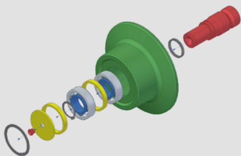
Kladka člankového dopravního pásu s maznicí
